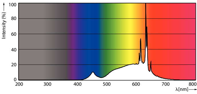
40W E26 A19 927 Frosted
